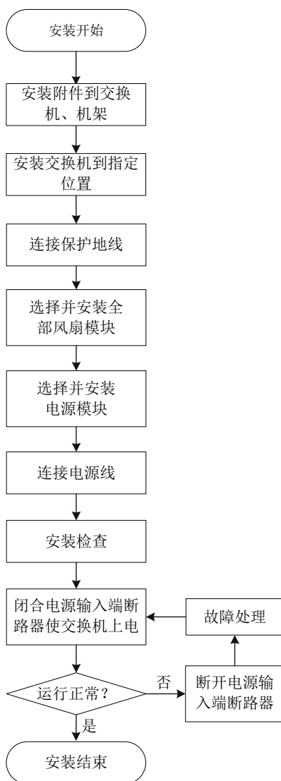
图2-1 交换机安装流程
