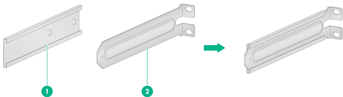
图2-7 1U 短滑道及滑道导轨示意图
