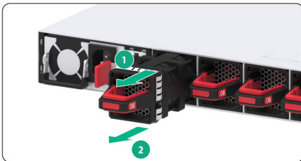
图2-17 风扇模块拆卸示意图
