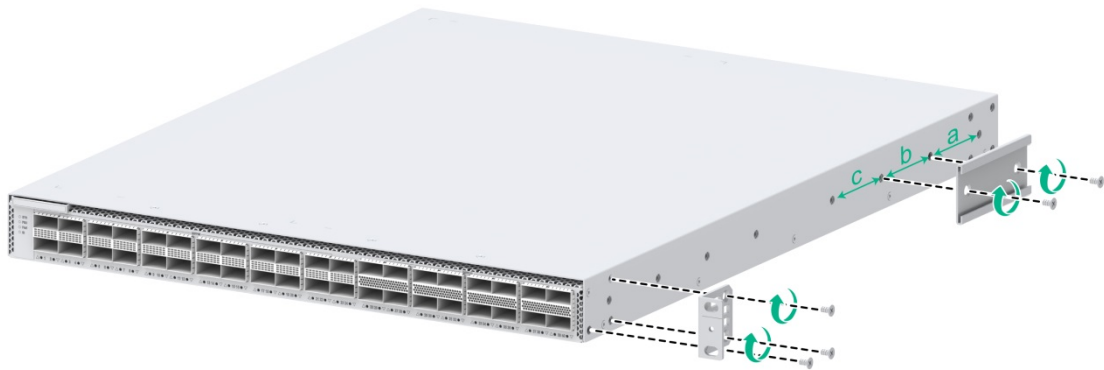
图2-11 安装挂耳和滑道导轨到 S9600XP-24B16DH-G 机箱（采用电源侧挂耳安装位）
