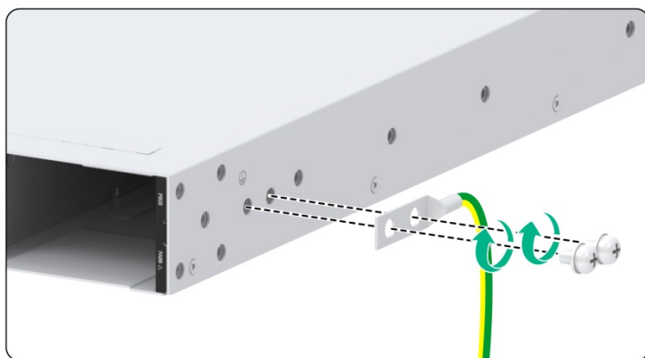
图2-12 安装接地线缆到 S9600XP-24B16DH-G 主用接地点示意图
