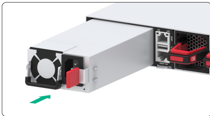
图2-20 电源模块安装示意图
