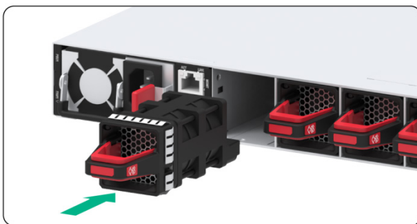
图2-16 风扇模块安装示意图
