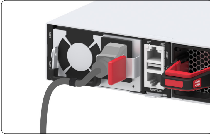
图2-24 PSR1300-12A-C-A-Z 交流电源线连接示意图
