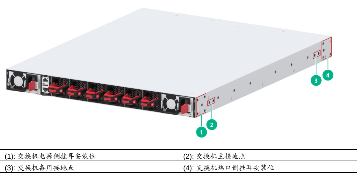
图2-9 S9600XP-24B16DH-G 挂耳安装位置、接地线缆连接位置
