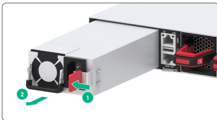
图2-22 拆卸电源模块示意图
