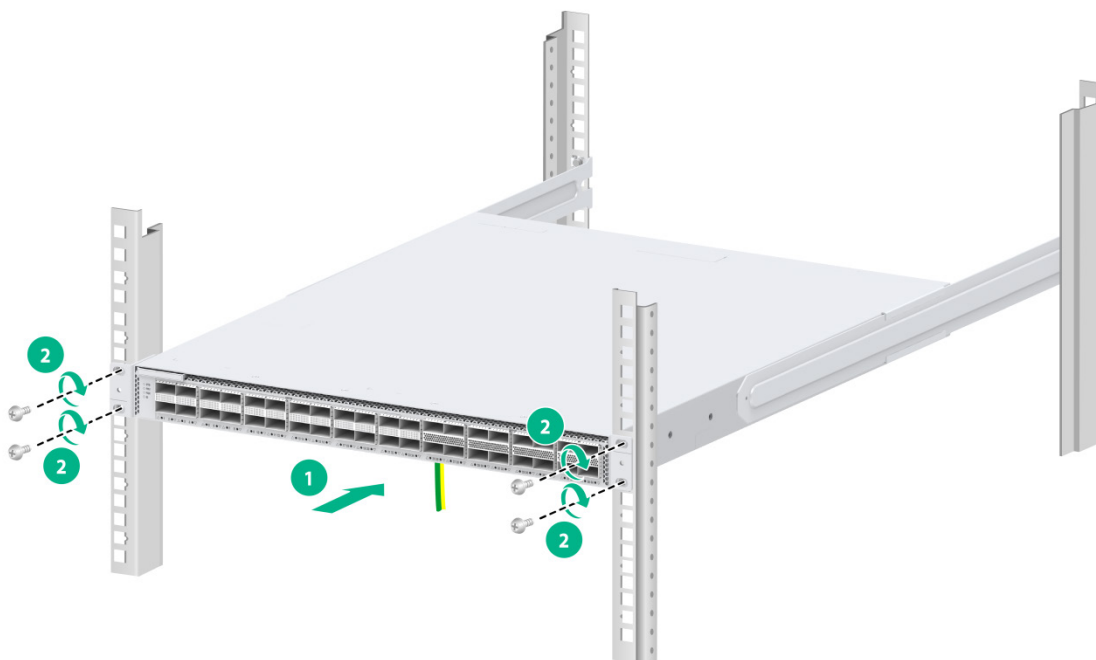
图2-14 安装 S9600XP-24B16DH-G 交换机到机柜示意图（挂耳安装在靠近端口侧）
