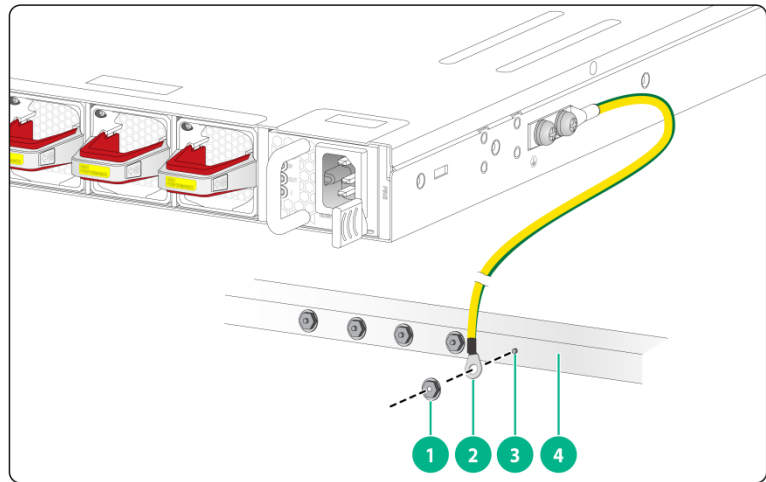
图2-2 连接接地线缆到接地排
