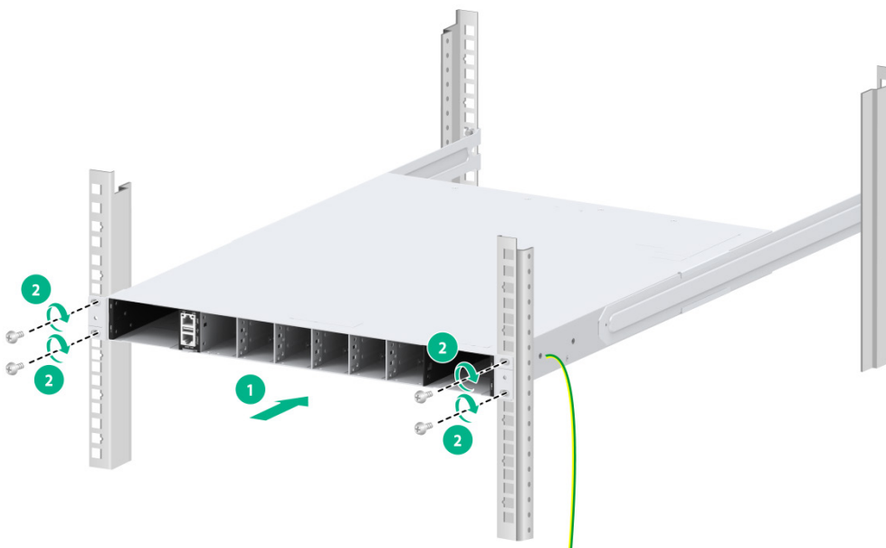
图2-15 安装 S9600XP-24B16DH-G 交换机到机柜示意图（挂耳安装在靠近电源侧）
