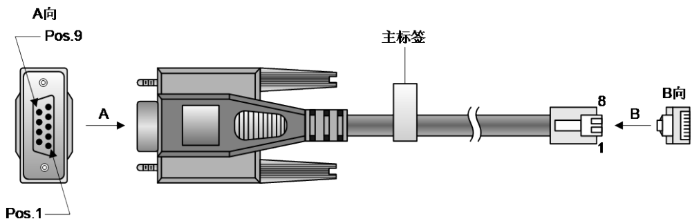
图3-2 串行配置口电缆示意图
