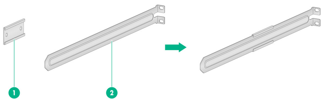
图2-8 1U 长滑道及滑道导轨示意图
